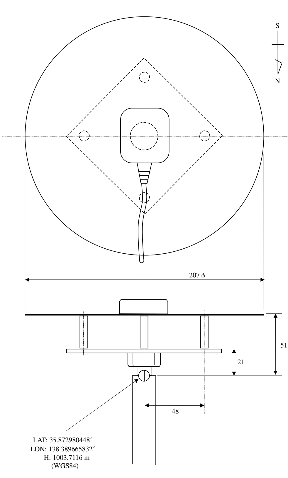
アンテナ評価用マウント+グラウンドプレーン
